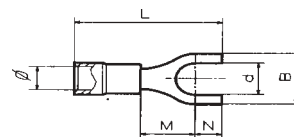
haarukkaliittimet
