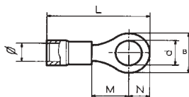
rengasliittimet
